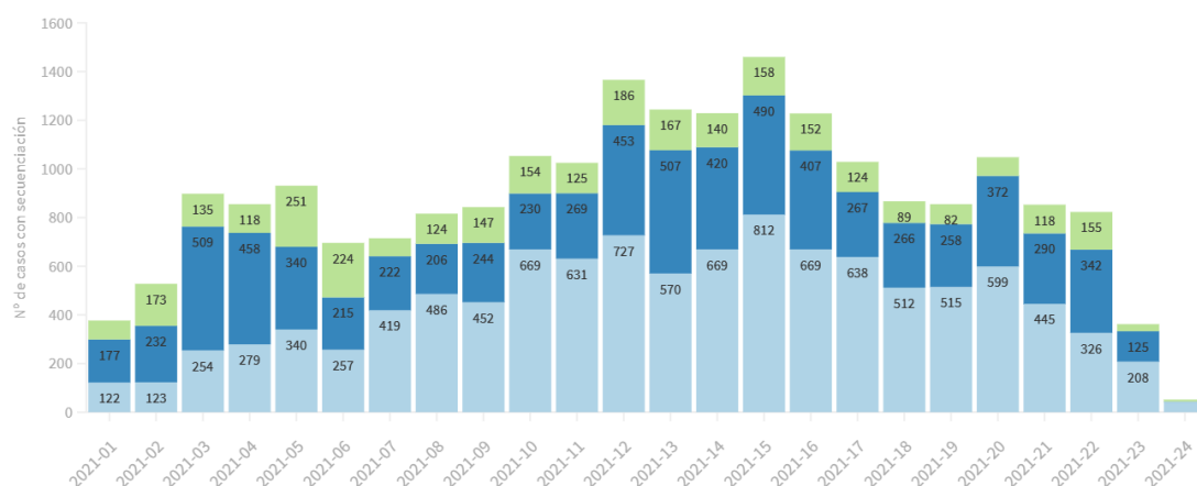
Figura 1. Número de casos secuenciados en España, en las semanas 1 a 24 (4 de enero a 20 de junio) de 2021.
