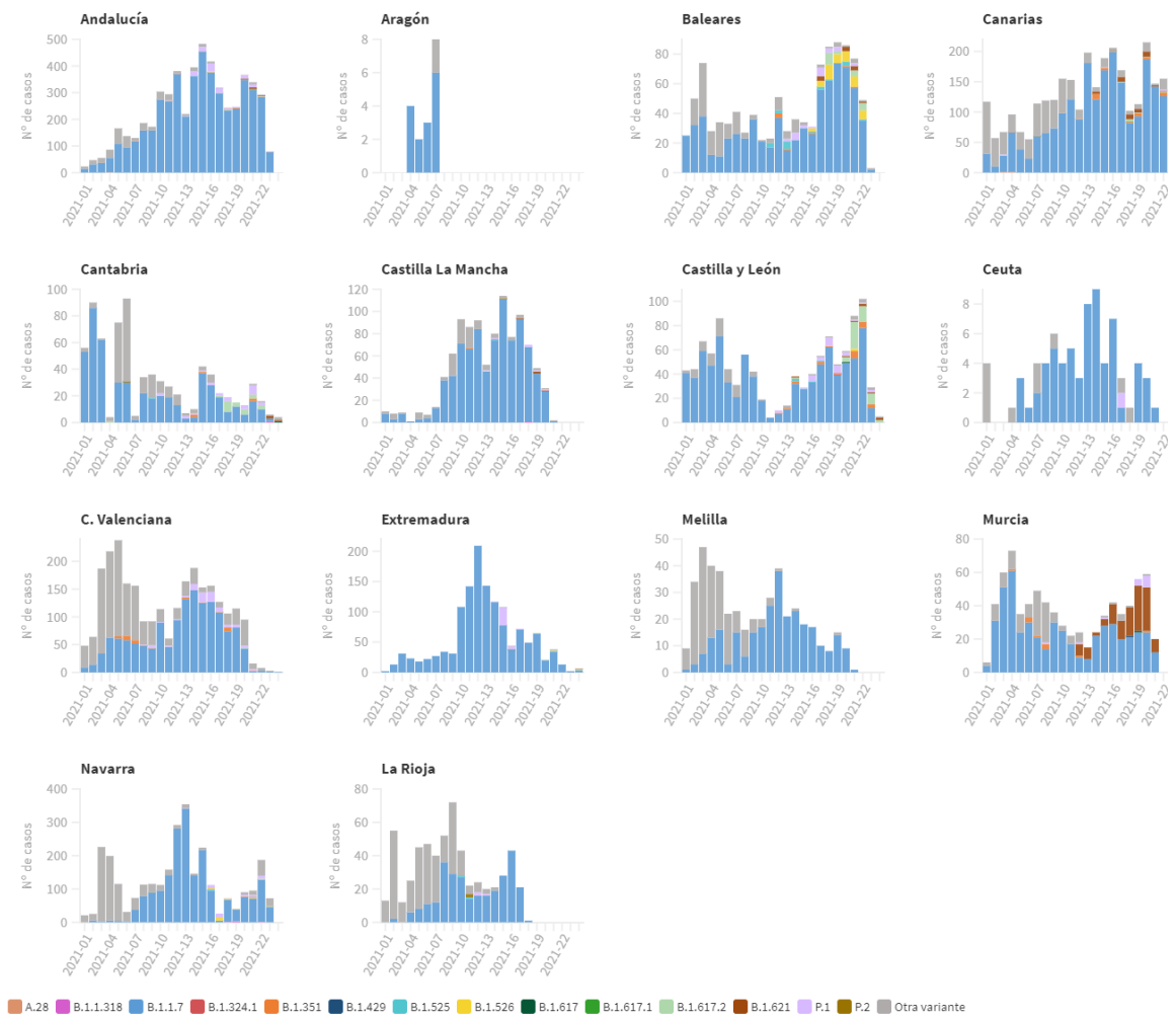
Figura 3: Número de secuencias totales por tipo de variante y semana para cada Comunidad Autónoma de la que se dispone de datos entre las semanas 1 y 24 (4 de enero a 20 de junio).
