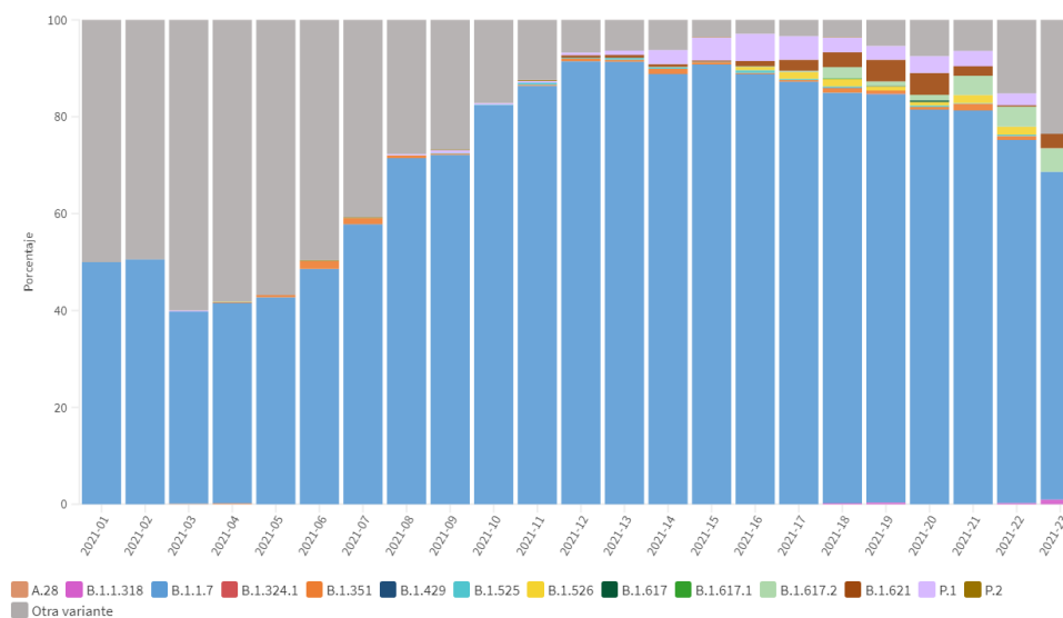
Figura 5: Porcentaje de cada tipo de variante por semana epidemiológica entre las semanas 1 y 23 (4 de enero a 13 de junio) de 2021 entre el número de muestras secuenciadas seleccionadas aleatoriamente.
